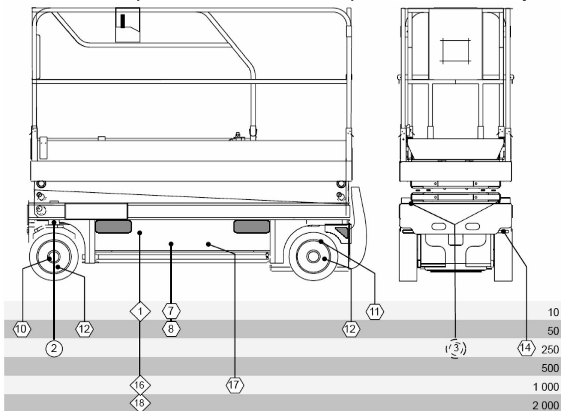
Рисунок 26. Схема технического обслуживания подъемника Compact 8.
