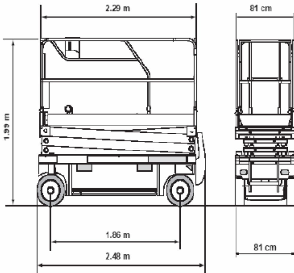
Рисунок 4. Габаритные размеры подъемника Compact 8.
