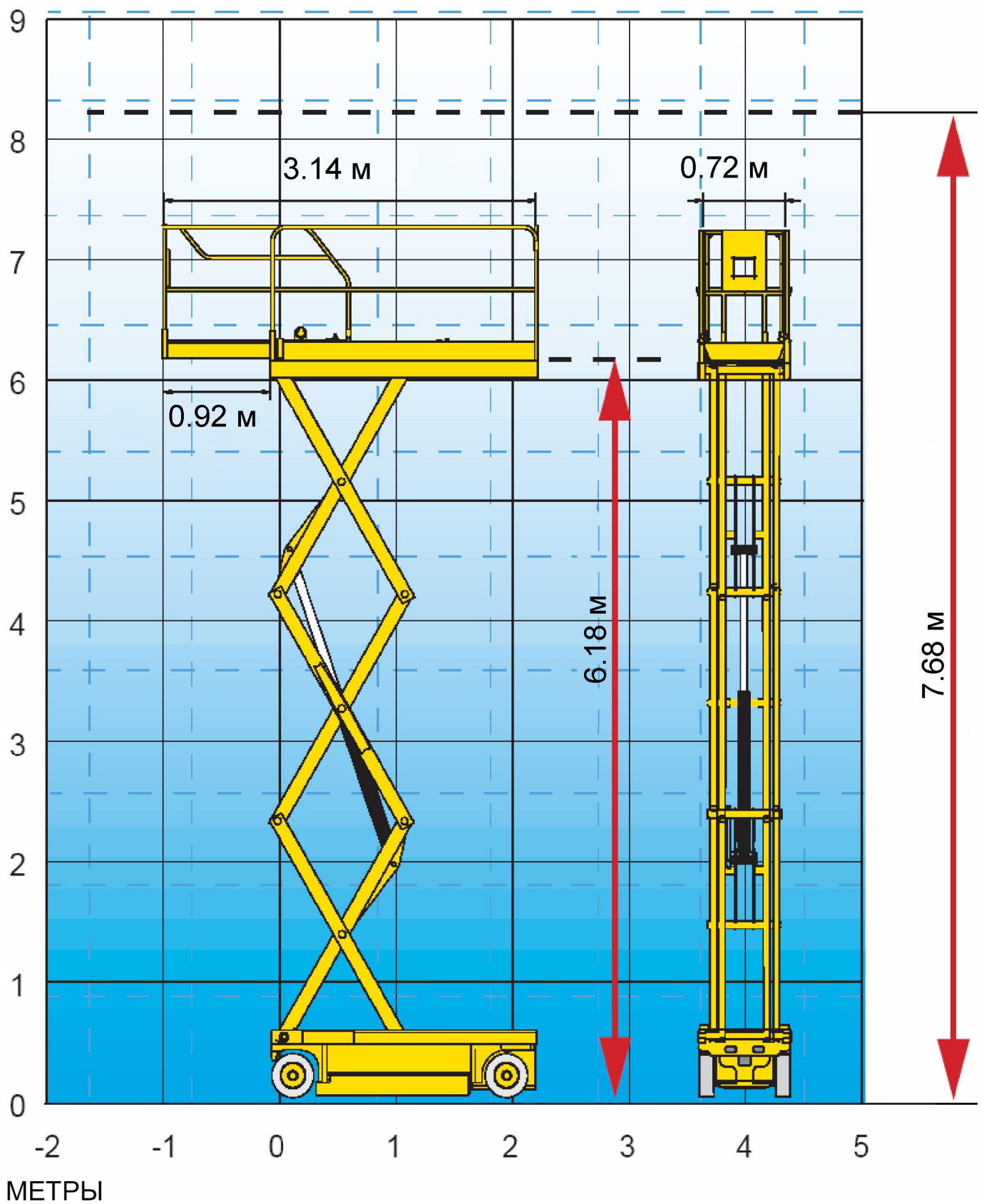
Рисунок 3. Рабочая зона подъемника Compact 8.
