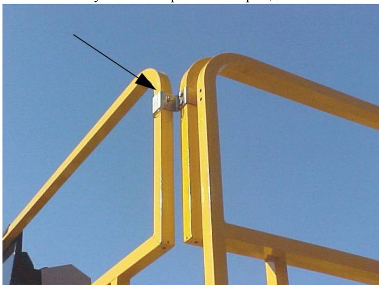
Рисунок 13. Закрепление ограждений.
