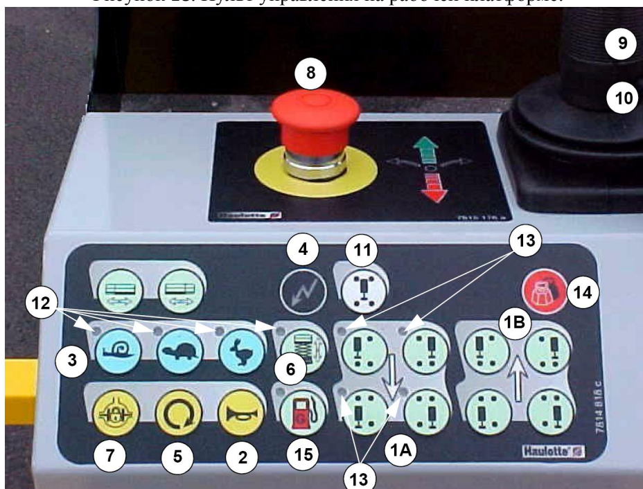
Рисунок 18. Пульта управления на рабочей платформе.
