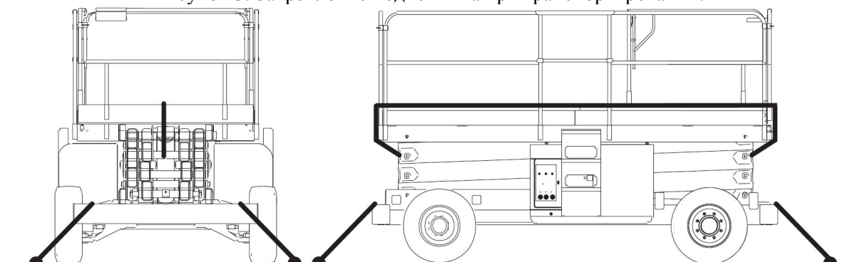
Рисунок 9. Закрепление подъемника при транспортировании.
