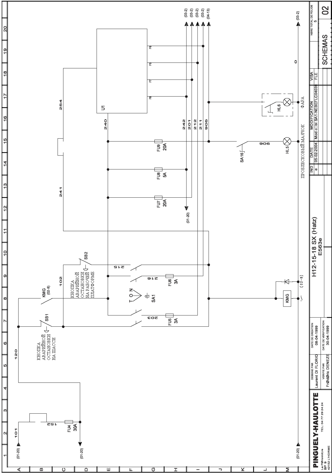
Рисунок 32. Гидравлическая схема подъемника Н 18 SX.
