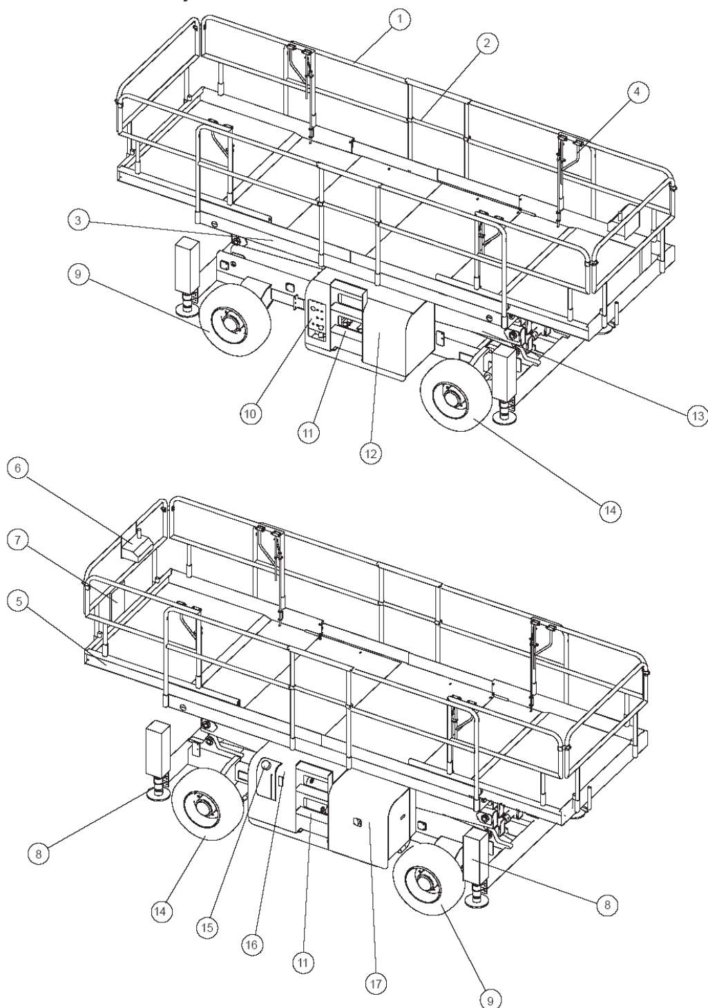
Рисунок 2. Основные элементы подъемника
