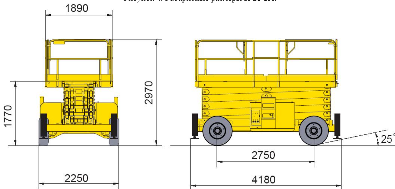
Рисунок 4. Габаритные размеры Н 18 SX.
