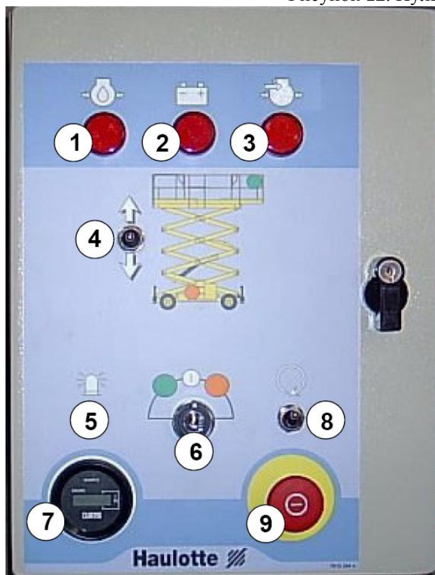
Рисунок 12. Пульт управления на шасси
