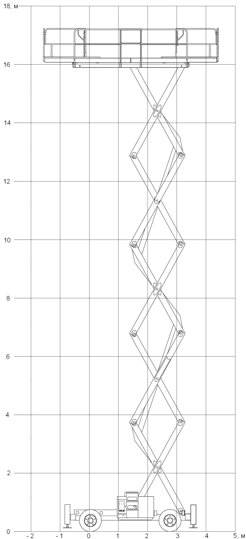
Рисунок 3. Рабочая зона подъемника Н 18 SX.
