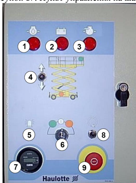
Рисунок 17. Пульт управления на шасси.
