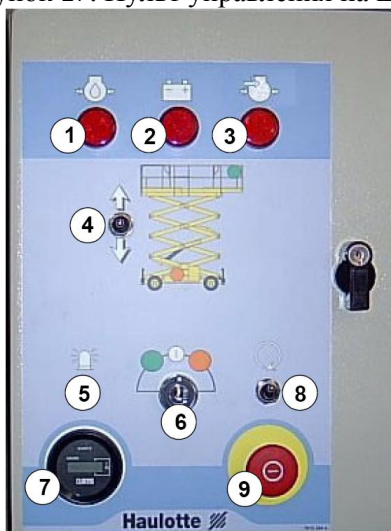
Рисунок 17. Пульт управления на шасси.
