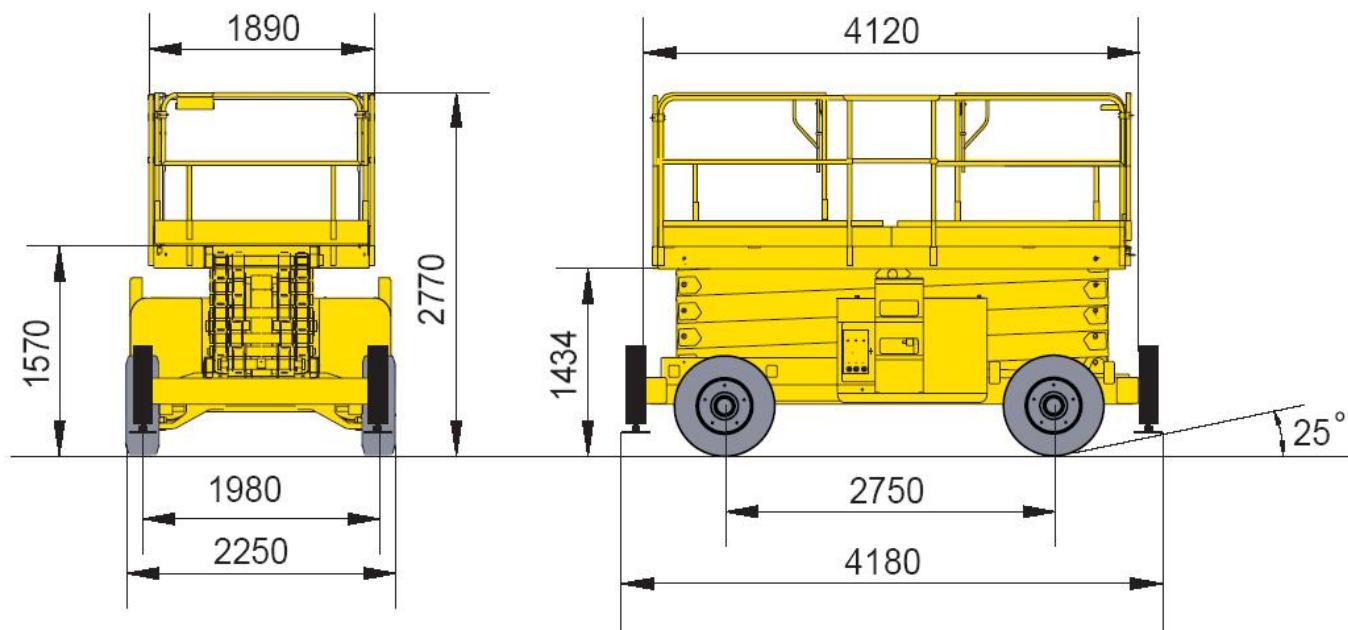
Рисунок 4. Габаритные размеры Н 15 SX.
