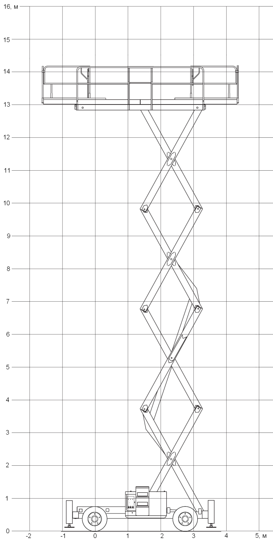
Рисунок 3. Рабочая зона подъемника Н 15 SX.
